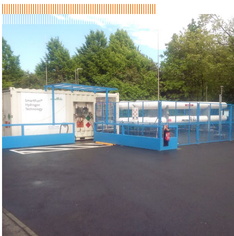
Wasserstofftankstelle im Daimler-Werk Düsseldorf
