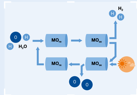
Prozessschema eines zweistufigen Kreisprozesses
