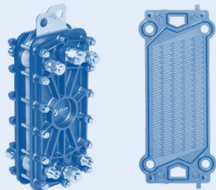
Beschichtete metallische Bipolarplatte mit Dichtung (links). 10-zelliger Stack mit metallischen Bipolarplatten und modifizierten Endplatten (rechts).
